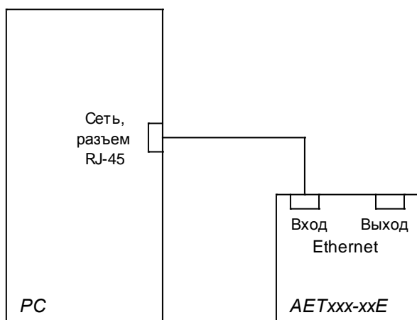
Подключение измерительного преобразователя АЕТ к интерфейсу сети компьютера.
