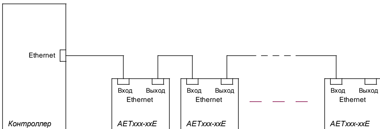
Подключение измерительных преобразователей АЕТ к интерфейсу Ethernet контроллера телемеханического комплекса.
