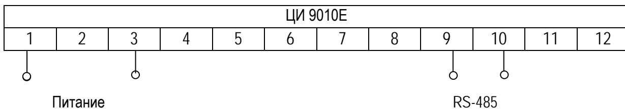
Рисунок Б.1 – Схема подключения ЦИ 9010Е
