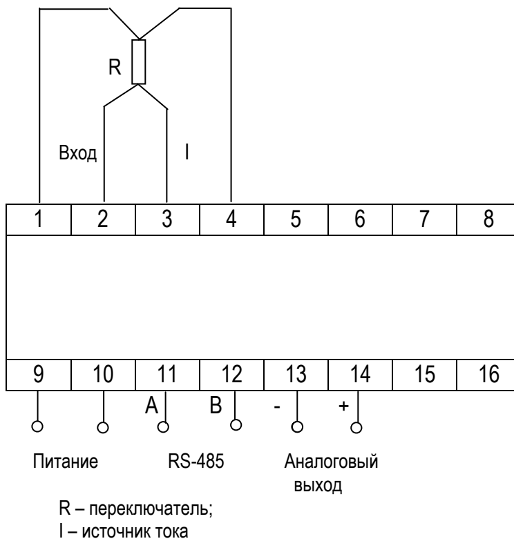
Рисунок А.1 – Схема электрическая подключения
