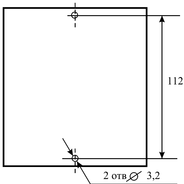
Рисунок А.2 - Установочные размеры преобразователя
