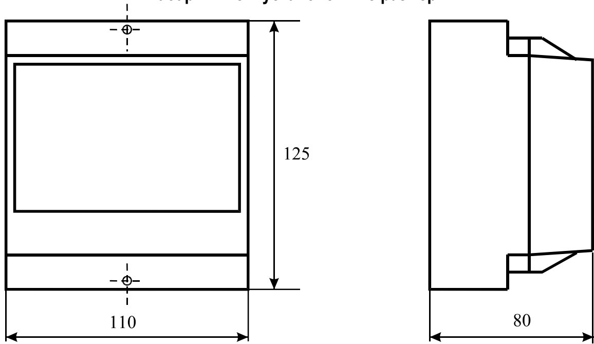
Рисунок А.1 - Габаритные размеры преобразователя
