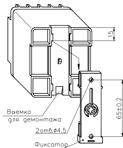
Рисунок В.2 Вариант крепления на панель
