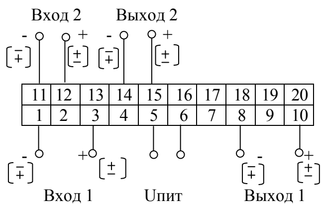
Рисунок А.3 - Схема электрическая подключений двухканальных ИП
