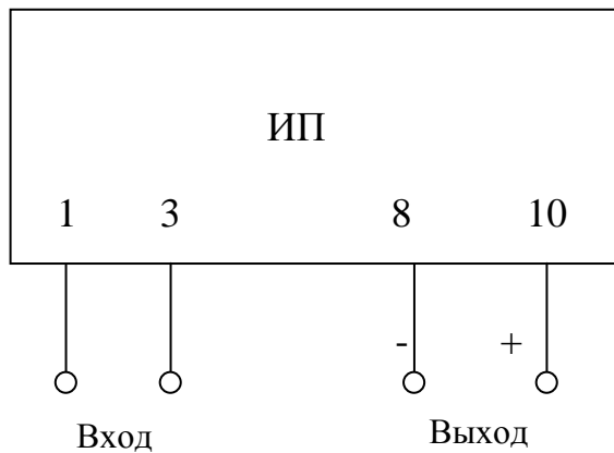
Рисунок А.2- Схема электрическая подключения
