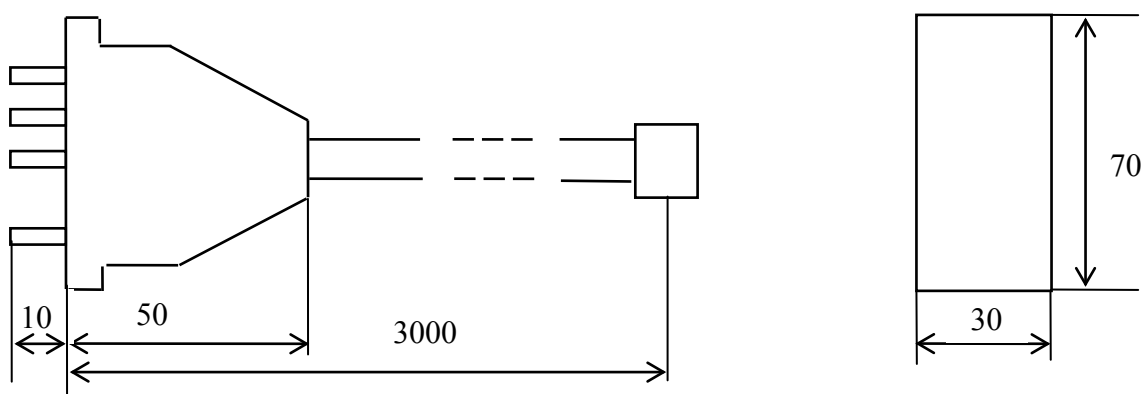
Рисунок Б.2 – Установочные размеры ИП
