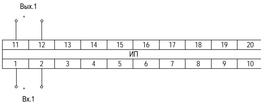
Рисунок Б.1- Схема электрическая подключений одноканальных ИП
