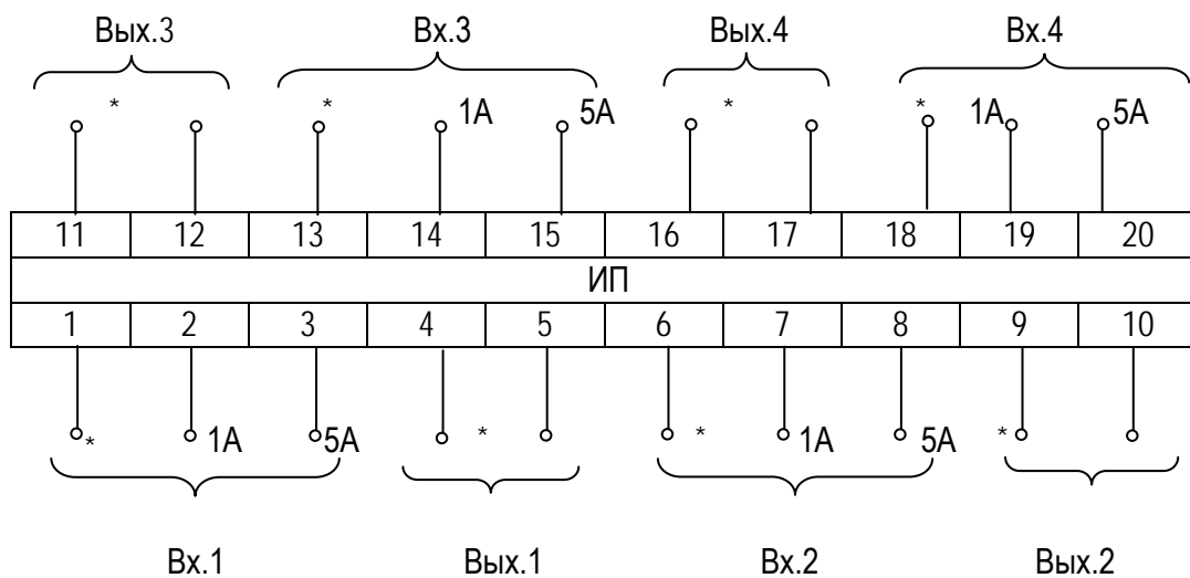
Рисунок Б.3- Схема электрическая подключений ИП Е 9527/22ЭС
