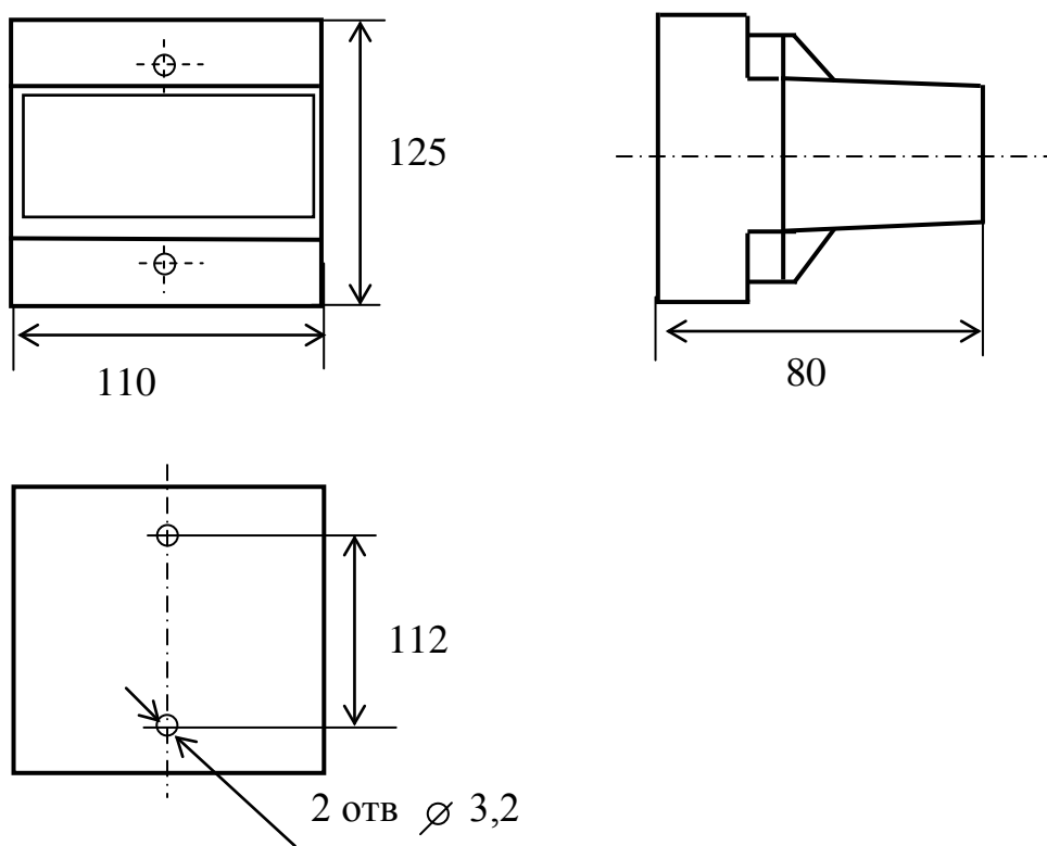
Рисунок А.1 – Габаритные и установочные размеры ИП
