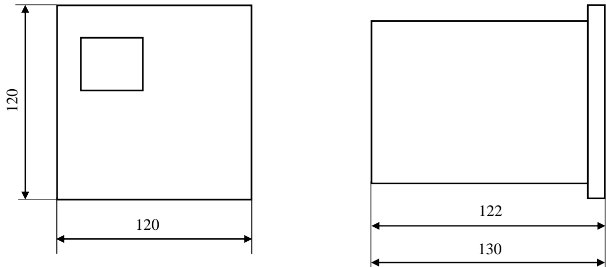
Рисунок А.1 – Габаритные размеры указателя
