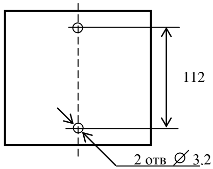
Рисунок Б.2 – Установочные размеры ЦП 9010/2
