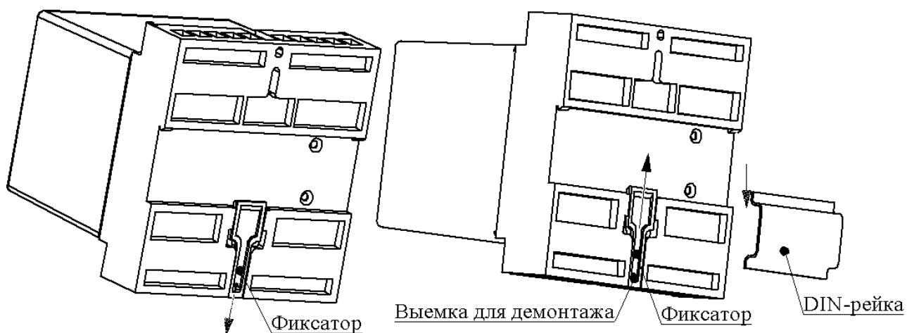
Рисунок А.2 – Схема установки на DIN-рейку
