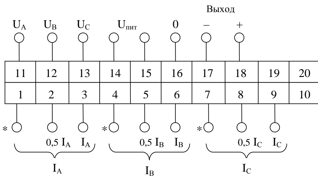
Рисунок А.4 – Схема подключения ИП E848M/3, E848M/4
