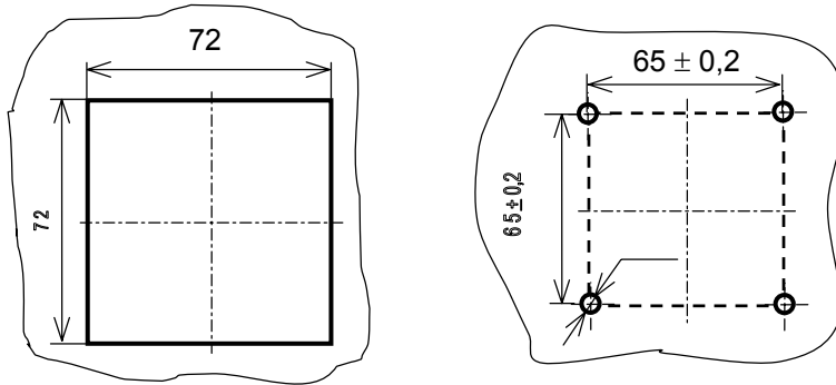
Рисунок В.1 – Разметка щита
