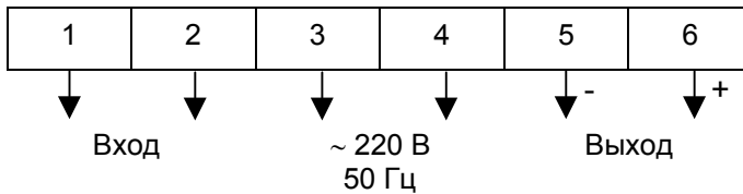
Рисунок В.3 – Схема электрическая подключения
