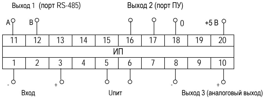
Рисунок Б.1 - Схема электрическая подключений ИП
