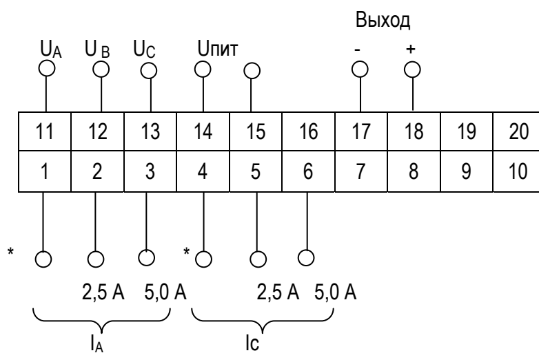
Рисунок А.2 – Схема подключения ИП Е 860/2ЭС, Е 860/4ЭС, Е 860/5ЭС, Е 860/7ЭС, Е 860/10ЭС
